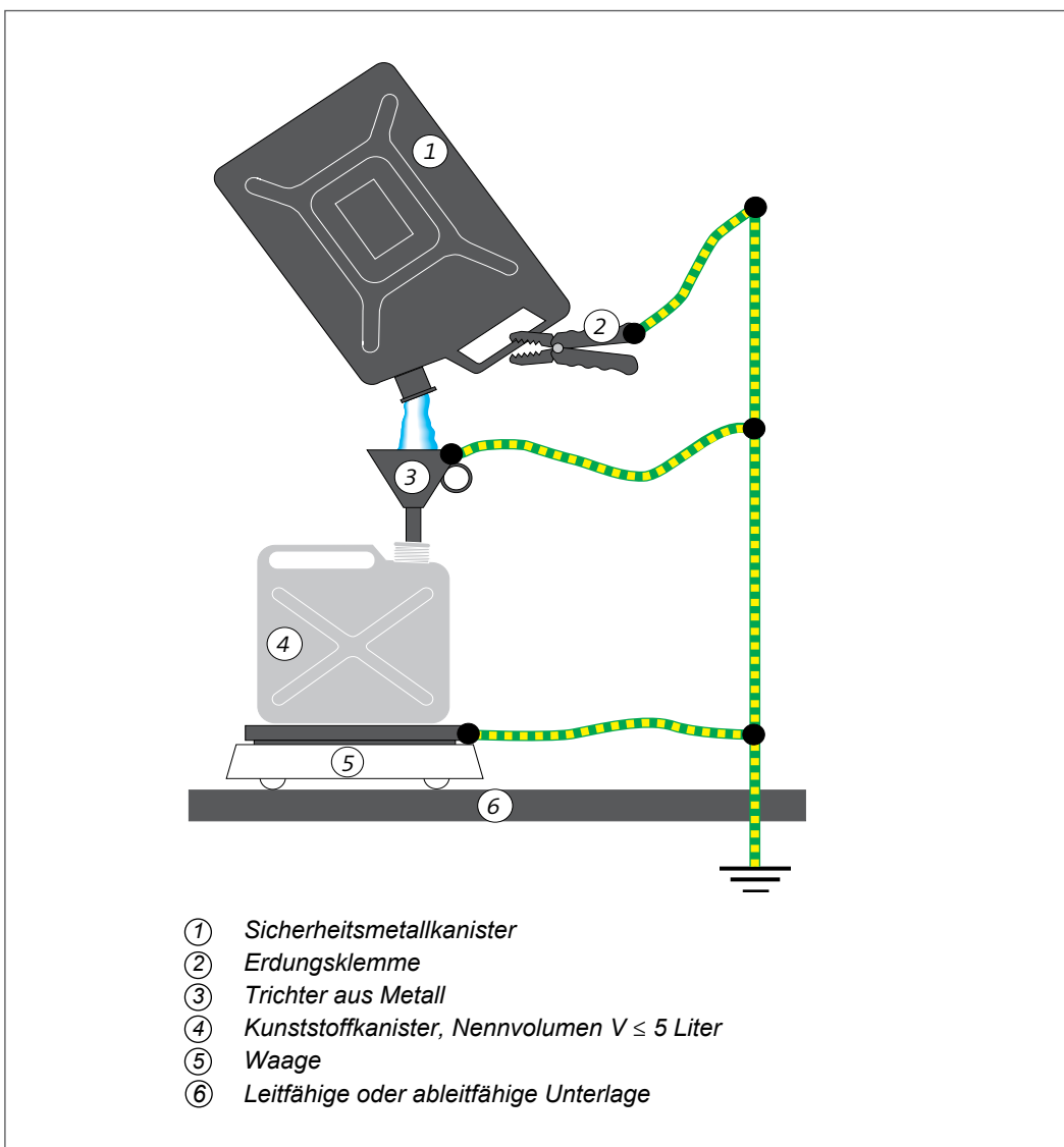
Beispiel 5: Befüllen kleiner Kunststoffkanister in Zone 1
