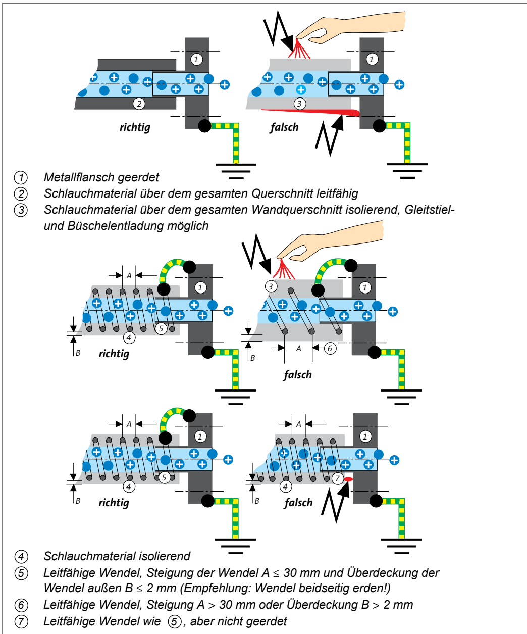
Beispiel 11: Schläuche zum pneumatischen Transport nicht brennbarer Schüttgüter durch Zone 1, die verursacht ist durch Gefahrstoffe der Explosionsgruppen IIA und IIB
