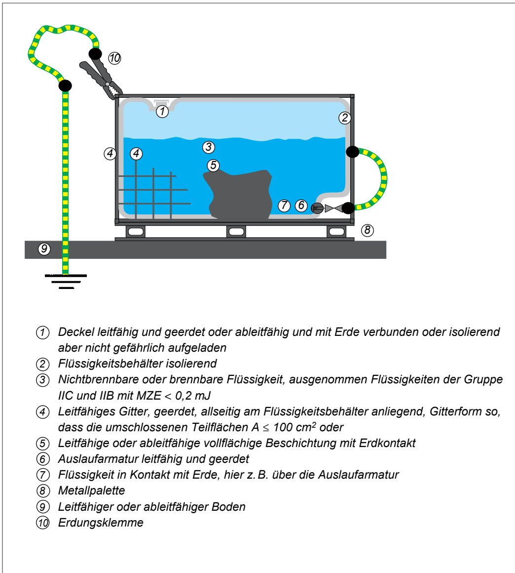
Beispiel 3: Befüllen und Entleeren von Rigid Intermediate Bulk Containern (RIBC) in Zone 1
