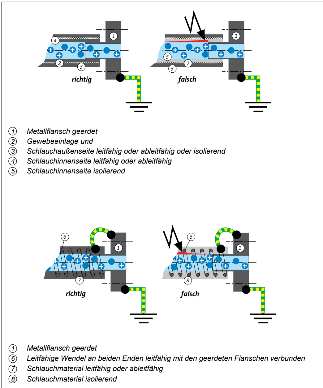
Beispiel 12: Schläuche zum pneumatischen Transport brennbarer Schüttgüter
