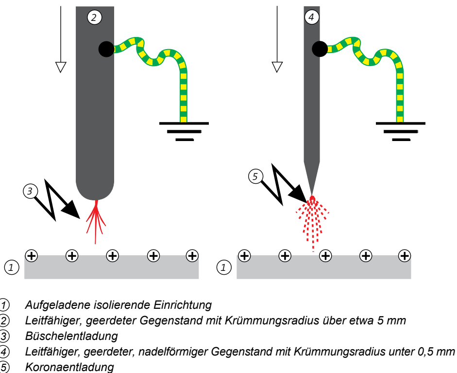
Beispiel 15: Büschelentladungen (links, vgl. Anhang A3.3) und Koronaentladungen (rechts, vgl. Anhang A3.2)
