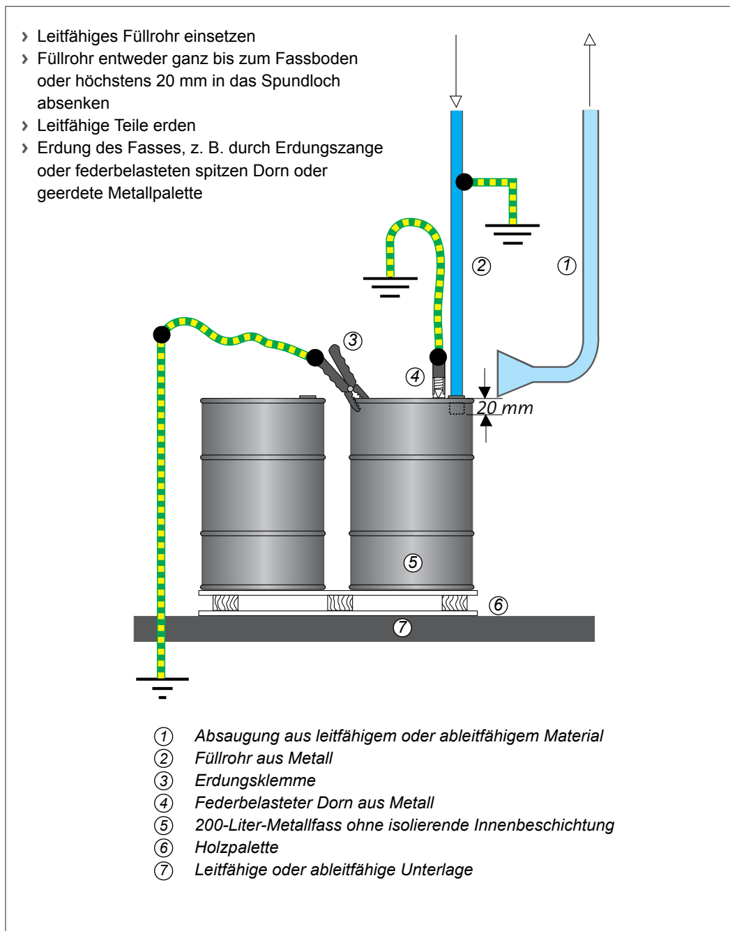
Beispiel 4: Befüllen von Fässern in Zone 1
